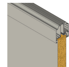
ISO-Paneel in thermisch getrennten Alu-Rahmen eingefasst.
